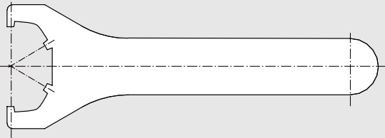
Spannschlüssel für Spannmutter ER 25-40/Wrench for locknuts ER 25-40
