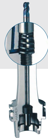
Vorspannfeder für Längeneinstellung Tension spring for length presetting
