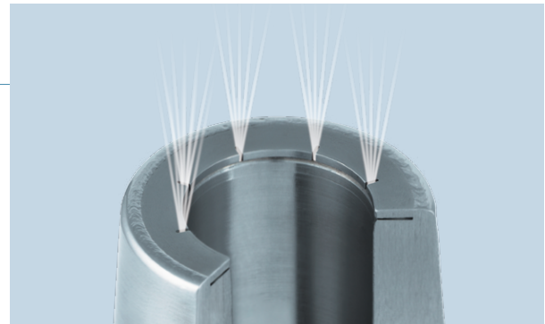
Optimierte Kühlmittelbohrung mit KSS-Austritt durch Schlitz Cool Flash System von HAIMER Optimized coolant bores with coolant outlet through slots Cool Flash by HAIMER
