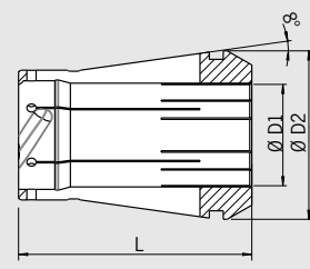
Spannzange Power Collet mit Safe-Lock™ Power Collet with Safe-Lock™
